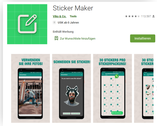
Abbildung 1: Beispiel-App „Sticker-Maker“
